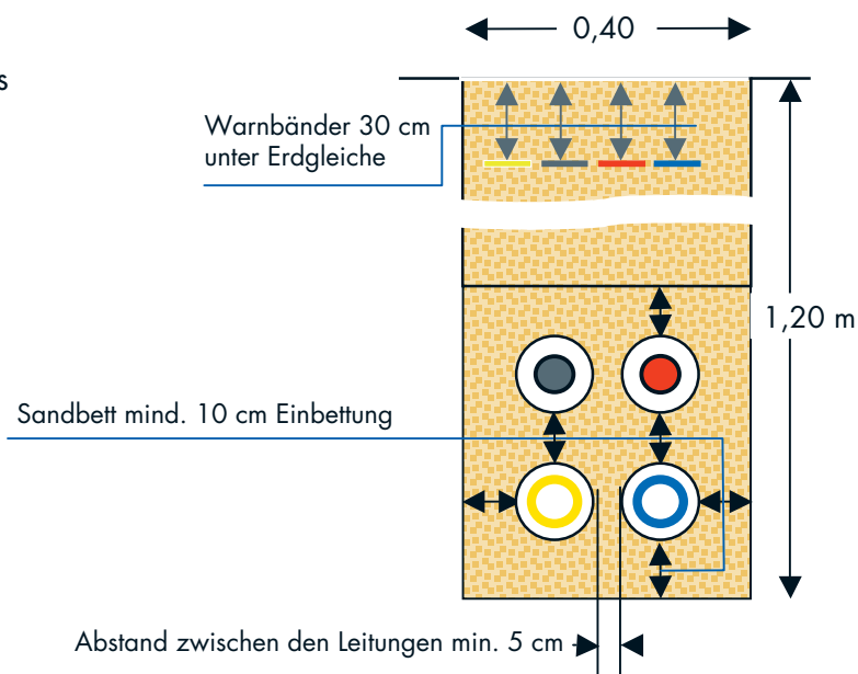
Grabenprofil Netzanschluss mit Schutzrohr
